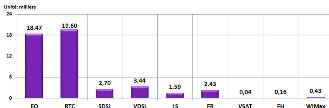
Fig19 : Répartition des abonnements data fixe autres que l'ADSL, box data et LTE-TDD par type de technologie fin août 2017.
